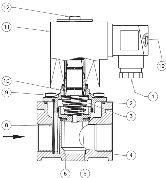
fig. 1 EW... (apertura rapida) EW... (fast opening) EW... (ouverture rapide) EW... (apertura rápida)
